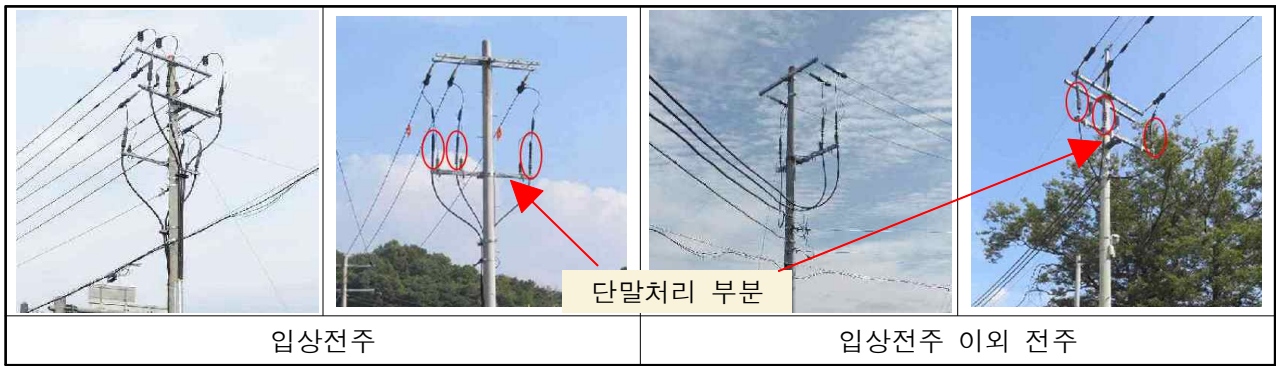
[그림 1] 케이블 단말처리 전주 사진
